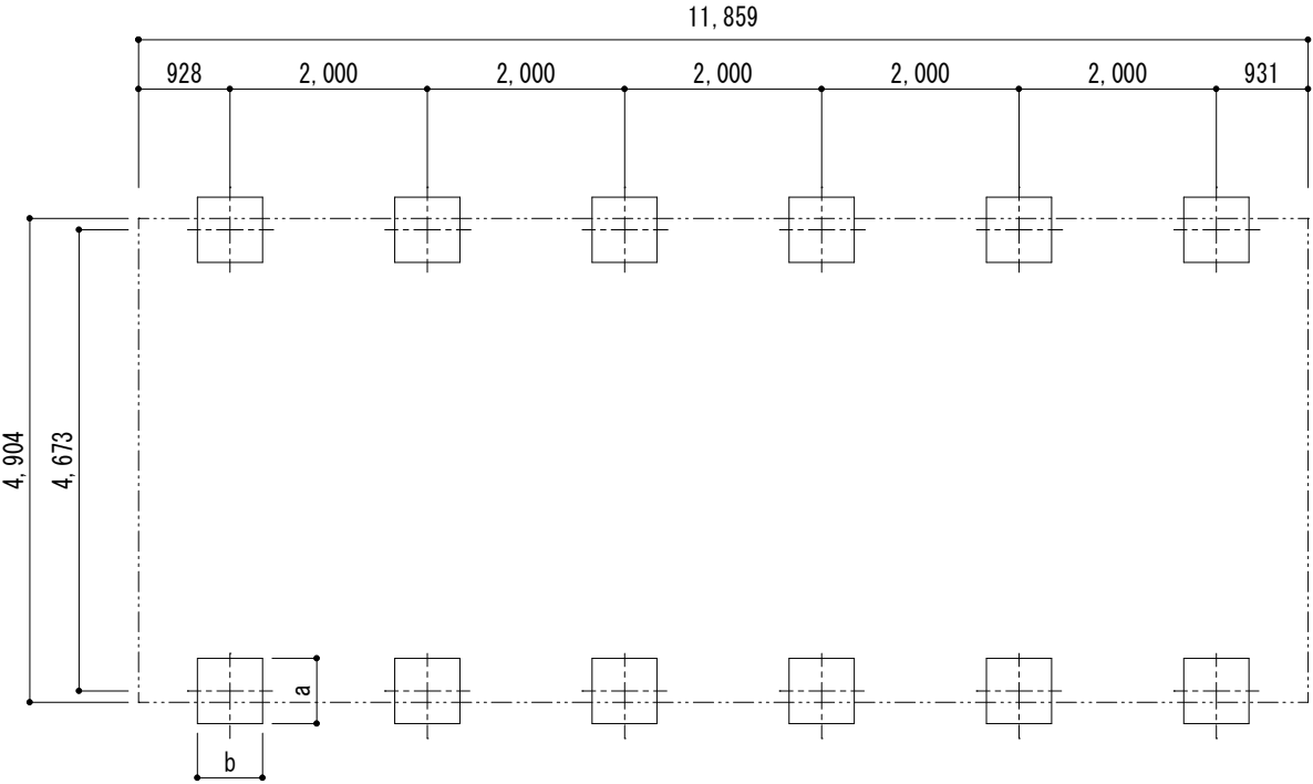
■基礎配置図
